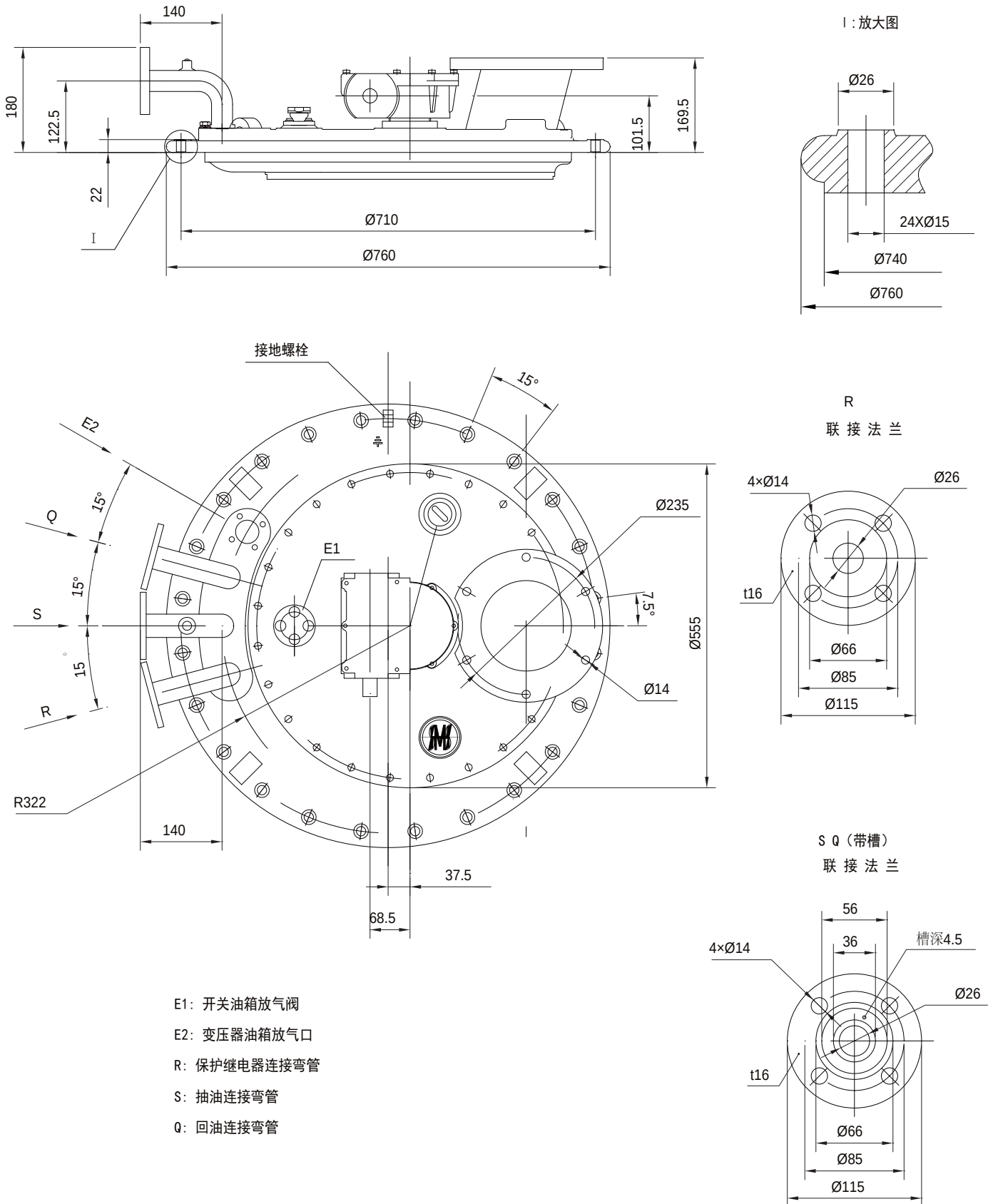
附图 21 CM 型有载开关带压力释放阀升高座安装法兰外形尺寸图
