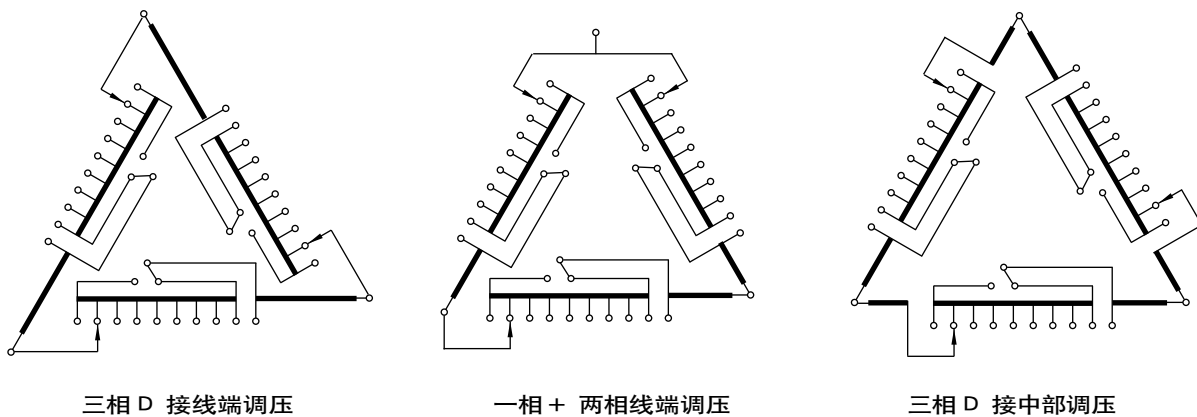
图 10 用于 D 接变压器绕组的基本接法
