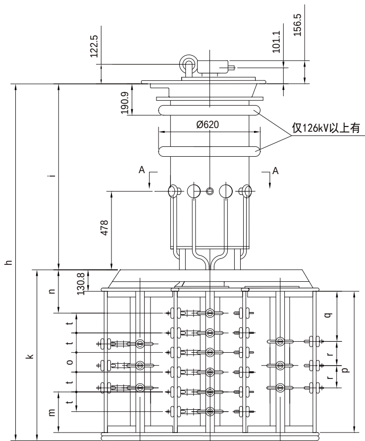
附图 34 CM | 1200/1500 多级开关外形尺寸图
