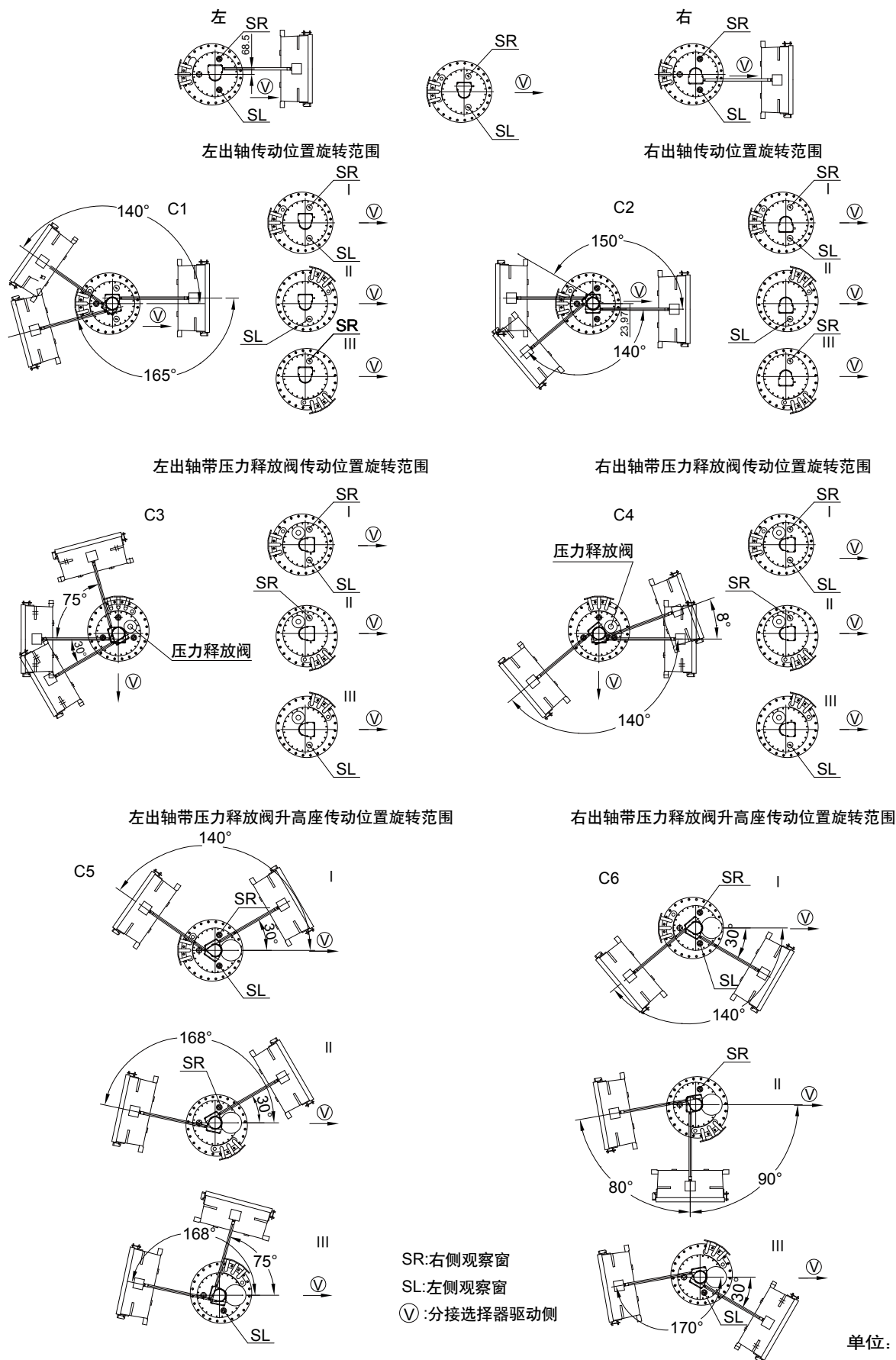
附图 22 齿轮机构传动轴位置布置图
