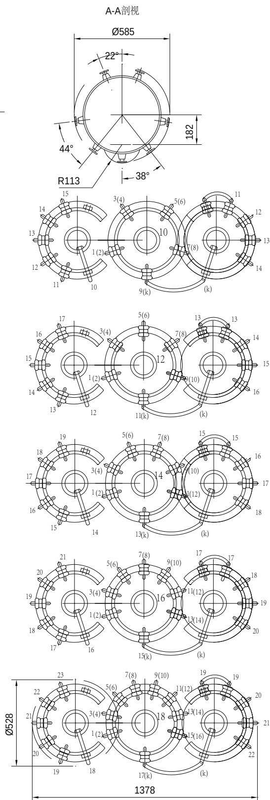
附图 34 CM | 1200/1500 多级开关外形尺寸图
