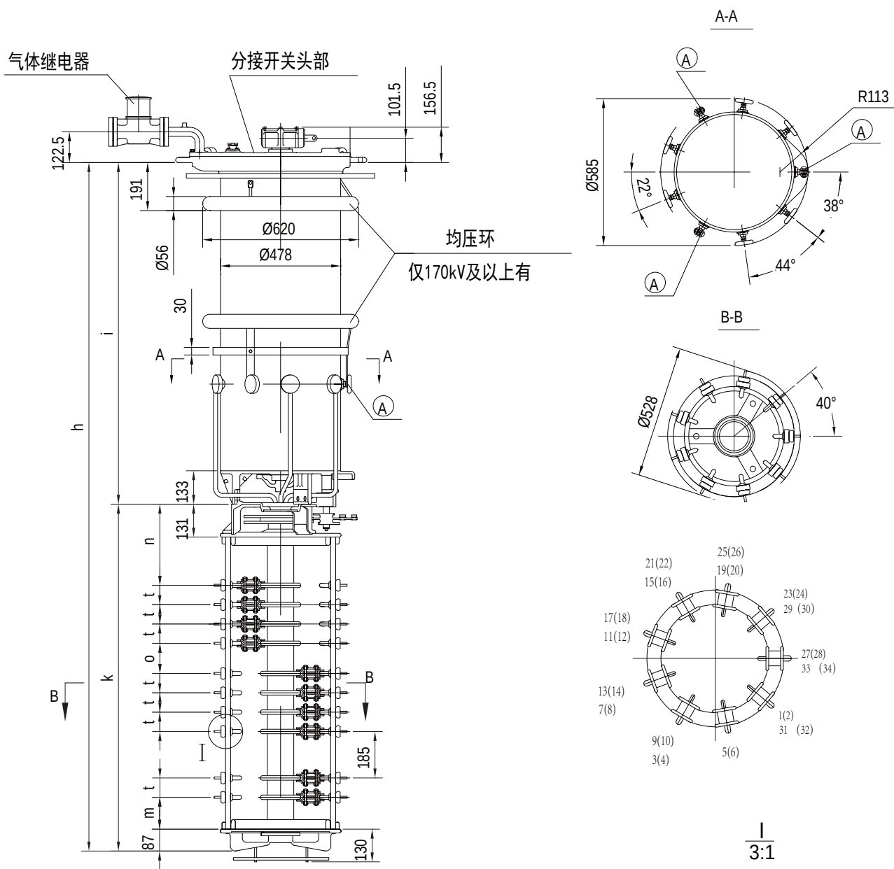
附图42 CM型有载开关 I 800 多级线性调开关外型尺寸图 (带电位电阻)
