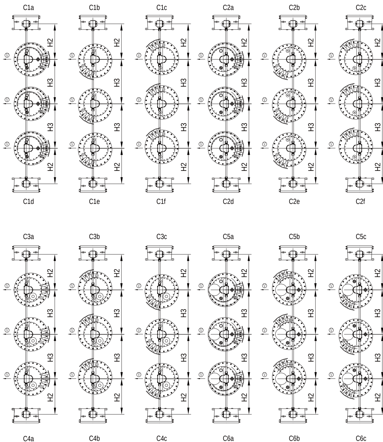
附图 23—1 CM 型有载开关布置图 1
