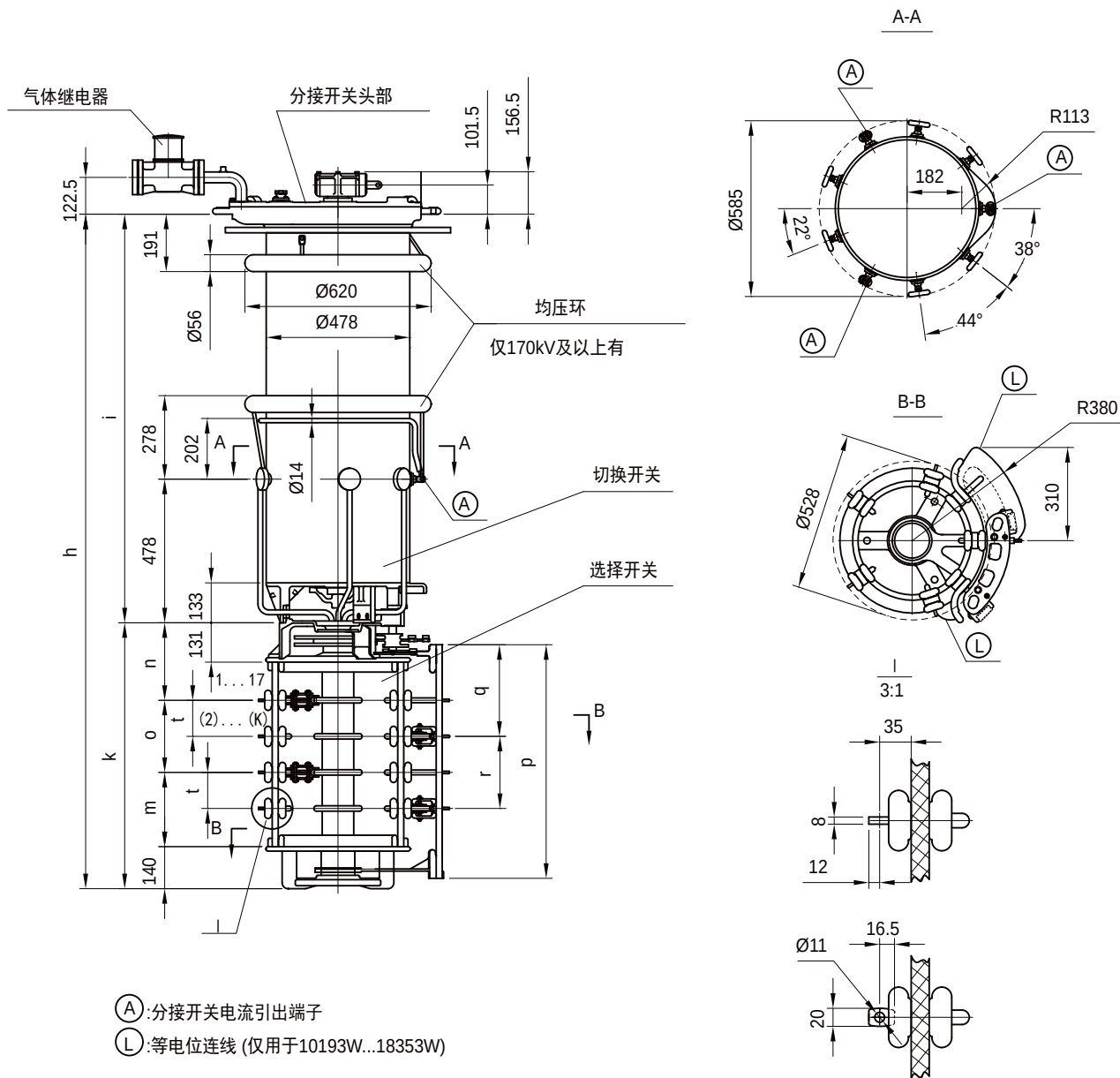
附图 5 CM 型有载开关 II 500/600 带极性选择器
