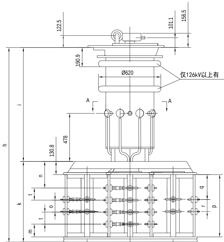
附图 33 CM I 800 多级开关外形尺寸图
