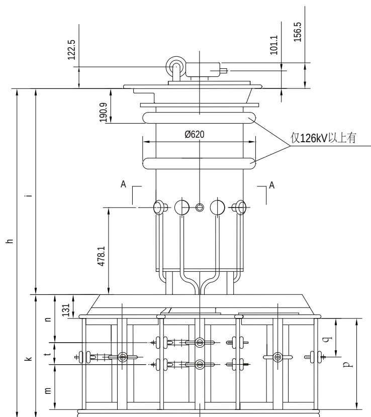
附图32 CM I 350/500/600多级开关外型尺寸图
