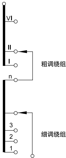
接线原理图
