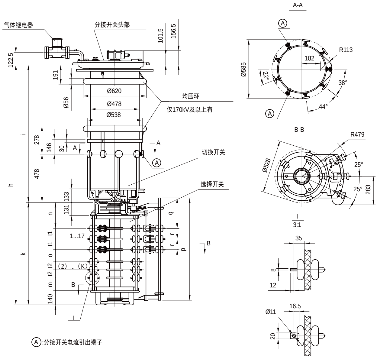
附图 15 CM 型有载开关 I 1200/1500 带粗细调选择器
