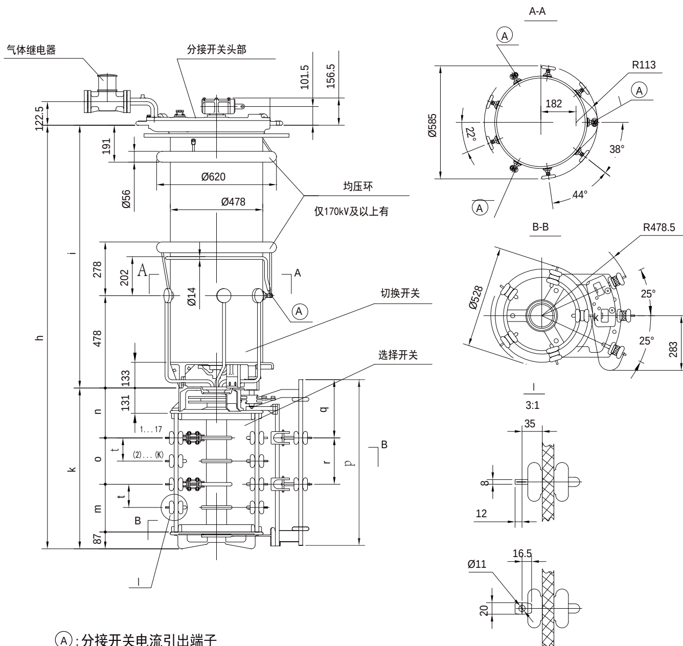
附图 6 CM 型有载开关 II 500/600 带粗细调选择器
