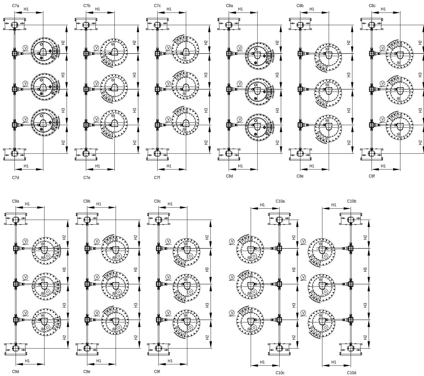
附图 23-2 CM 型有载开关布置图 2
