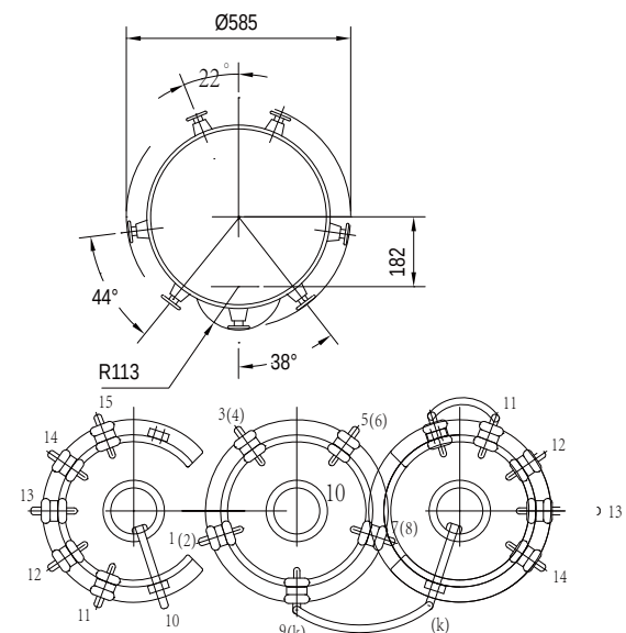
A-A剖视
