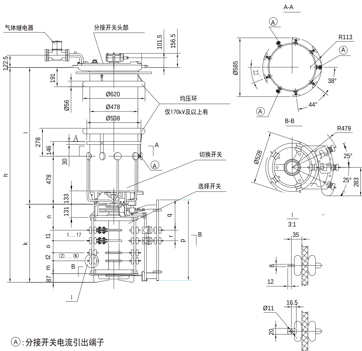
附图 12 CM 型有载开关 I 800 带粗细调选择器
