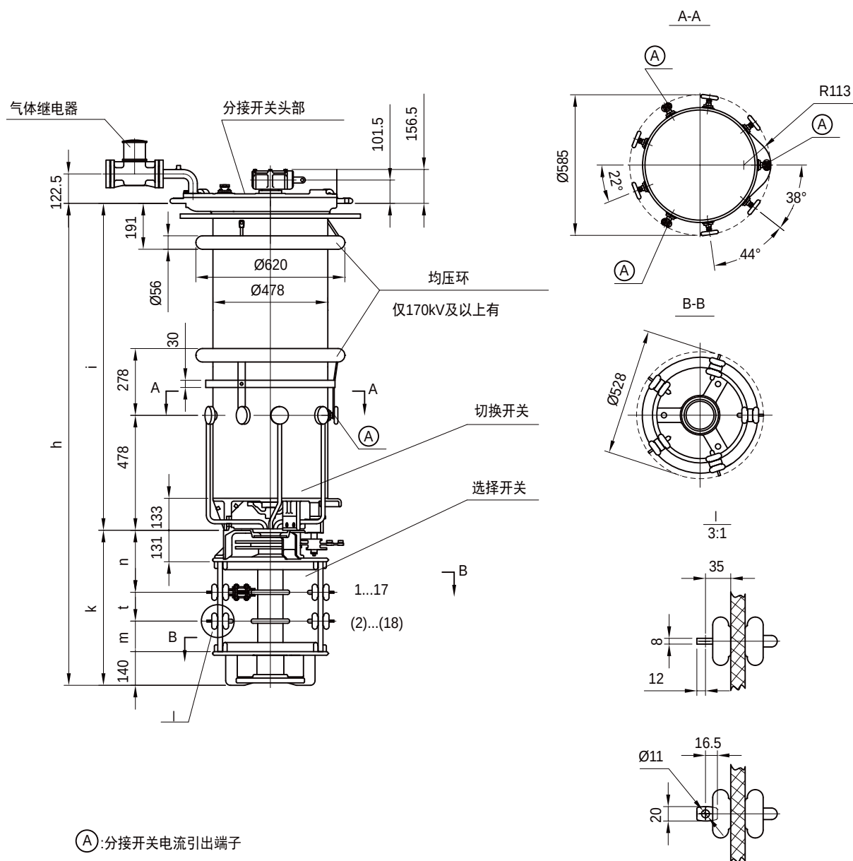
附图 7 CM 型有载开关 I 500/600 不带极性选择器
