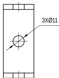
附图 28 CM 型有载开关 I 800/ I 1200/ I 1500 分接选择器 触头端子并联联接片尺寸图
