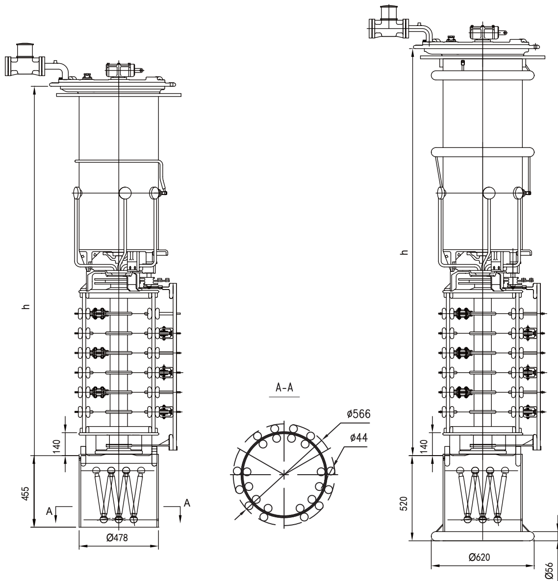
Um≤126kV外形尺寸图
