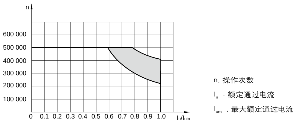
图6 平均负载下电弧触头的平均预期电气寿命
