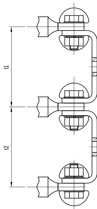
CM型 I 1200/1500触头端子联接图
