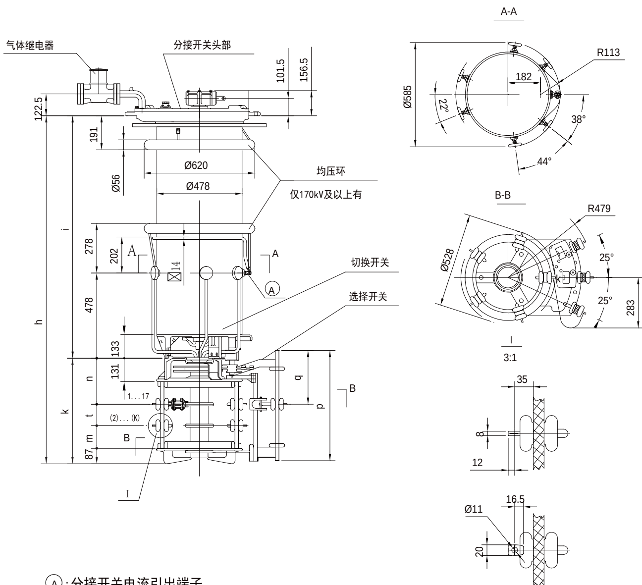
附图 9 CM 型有载开关 I 500/600 带粗细调选择器
