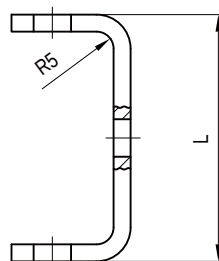
附图 28 CM 型有载开关 I 800/ I 1200/ I 1500 分接选择器 触头端子并联联接片尺寸图
