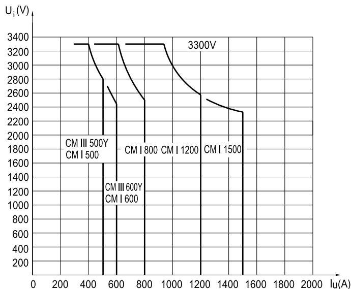
图 5 CM 型分接开关额定级容量
