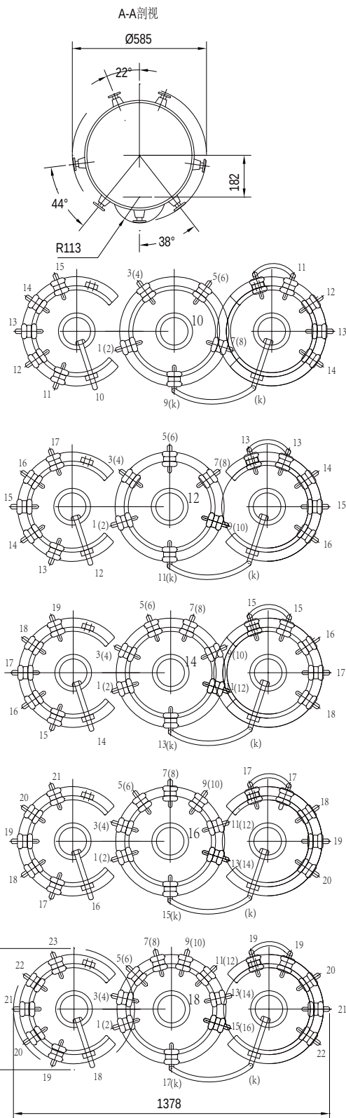
附图 33 CM I 800 多级开关外形尺寸图
