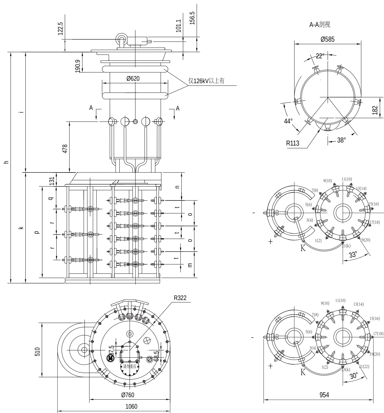
附图35 CM III 350Y/500Y/600Y 多级正反调开关外形尺寸图
