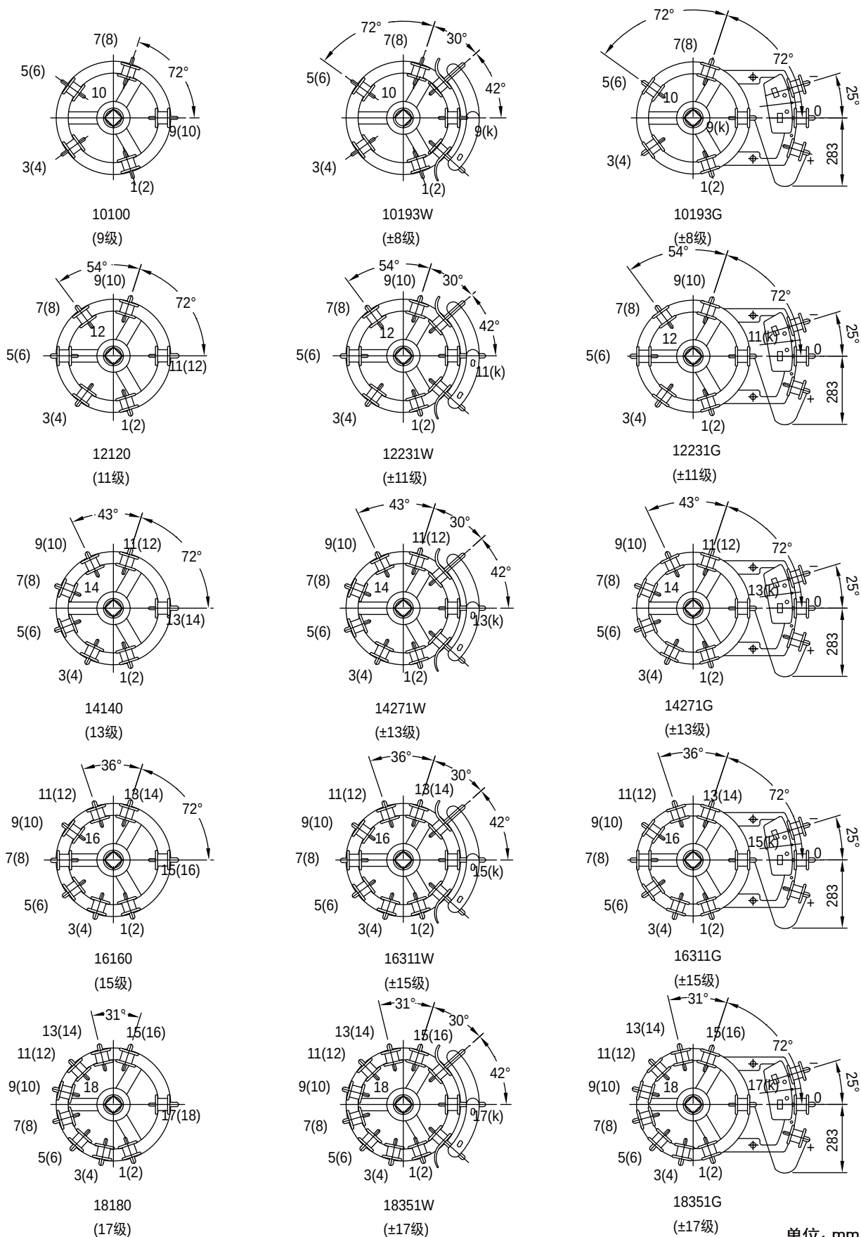
附图 18 CM 型有载开关触头排列布置示意图
