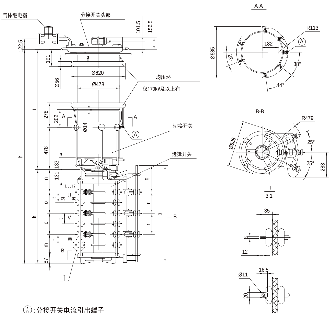
附图 3 CM 型有载开关 III 500Y/600Y 带粗细调选择器
