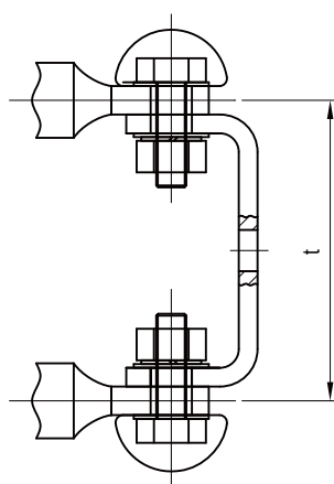
CM型 I 800触头端子联接图
