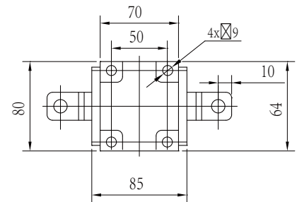
中间支撑盒外型尺寸图
