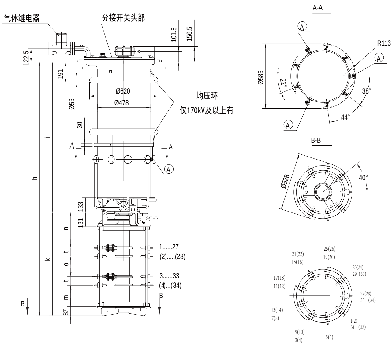
附图39 CM型有载开关 I 500/600 多级线性调选择器
