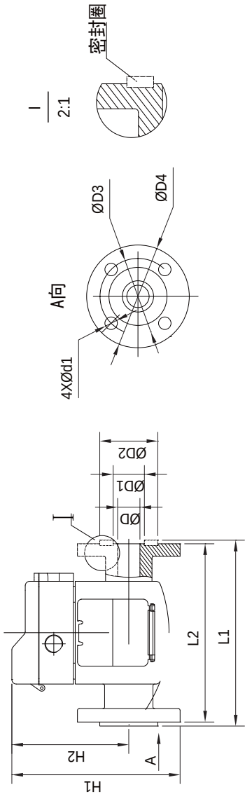
附图29 气体继电器的外形及安装尺寸图
