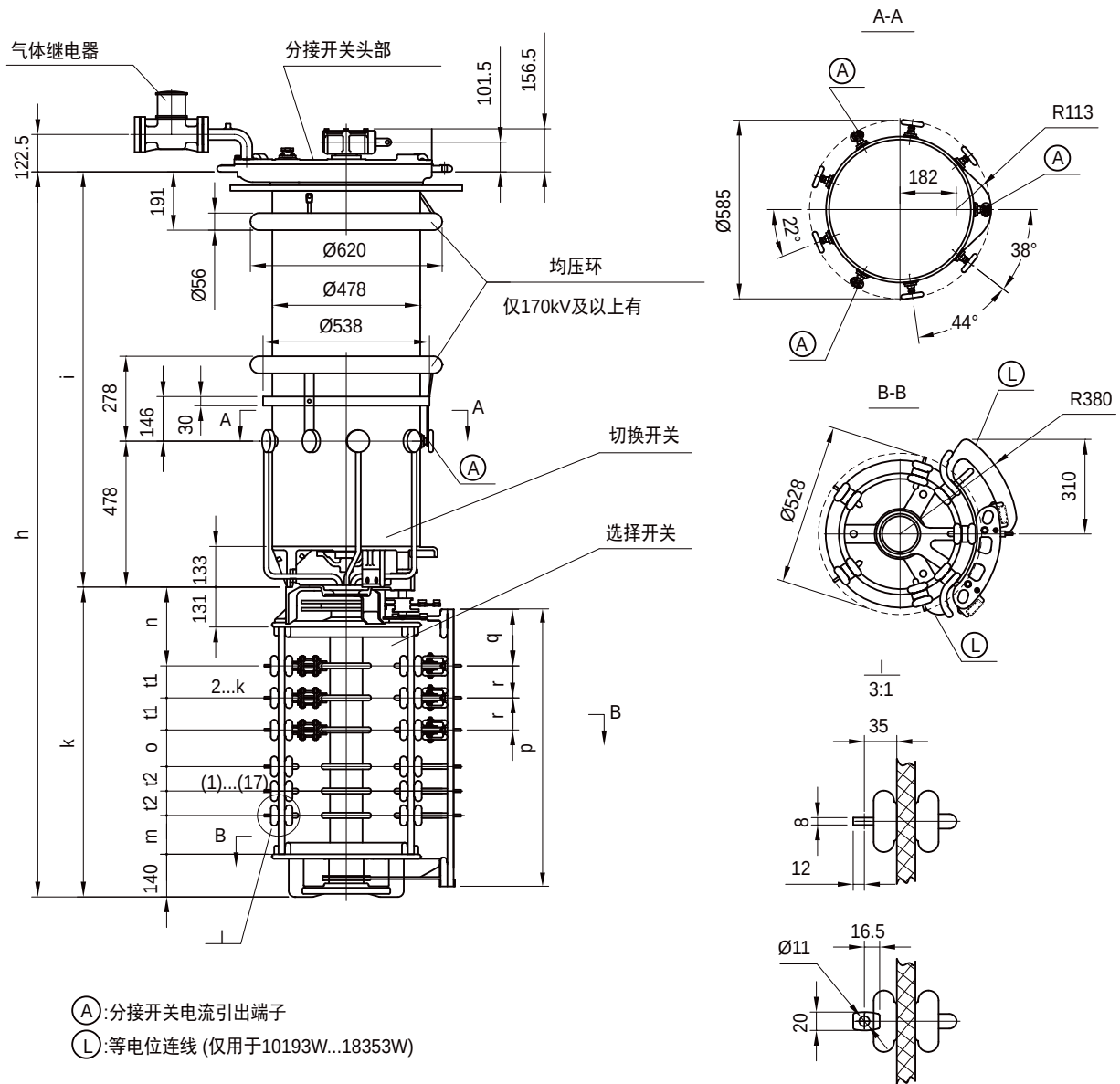
附图 14 CM 型有载开关 I 1200/1500 带极性选择器
