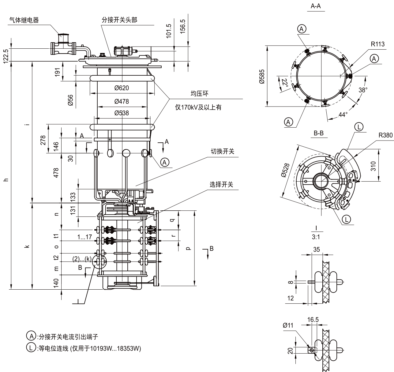
附图 11 CM 型有载开关 I 800 带极性选择器
