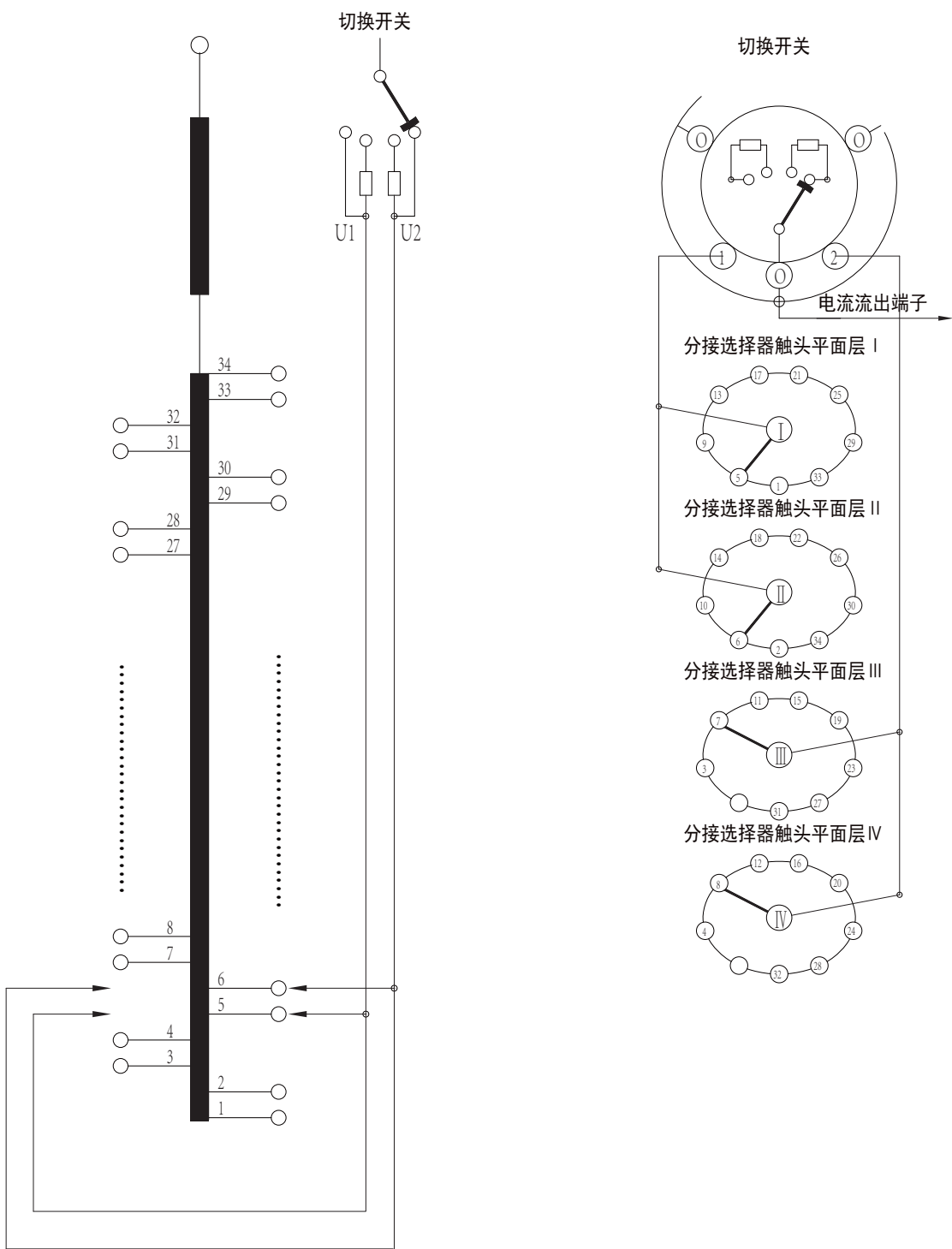
附图77 CM型有载开关工作位置表和接线图（36340）
