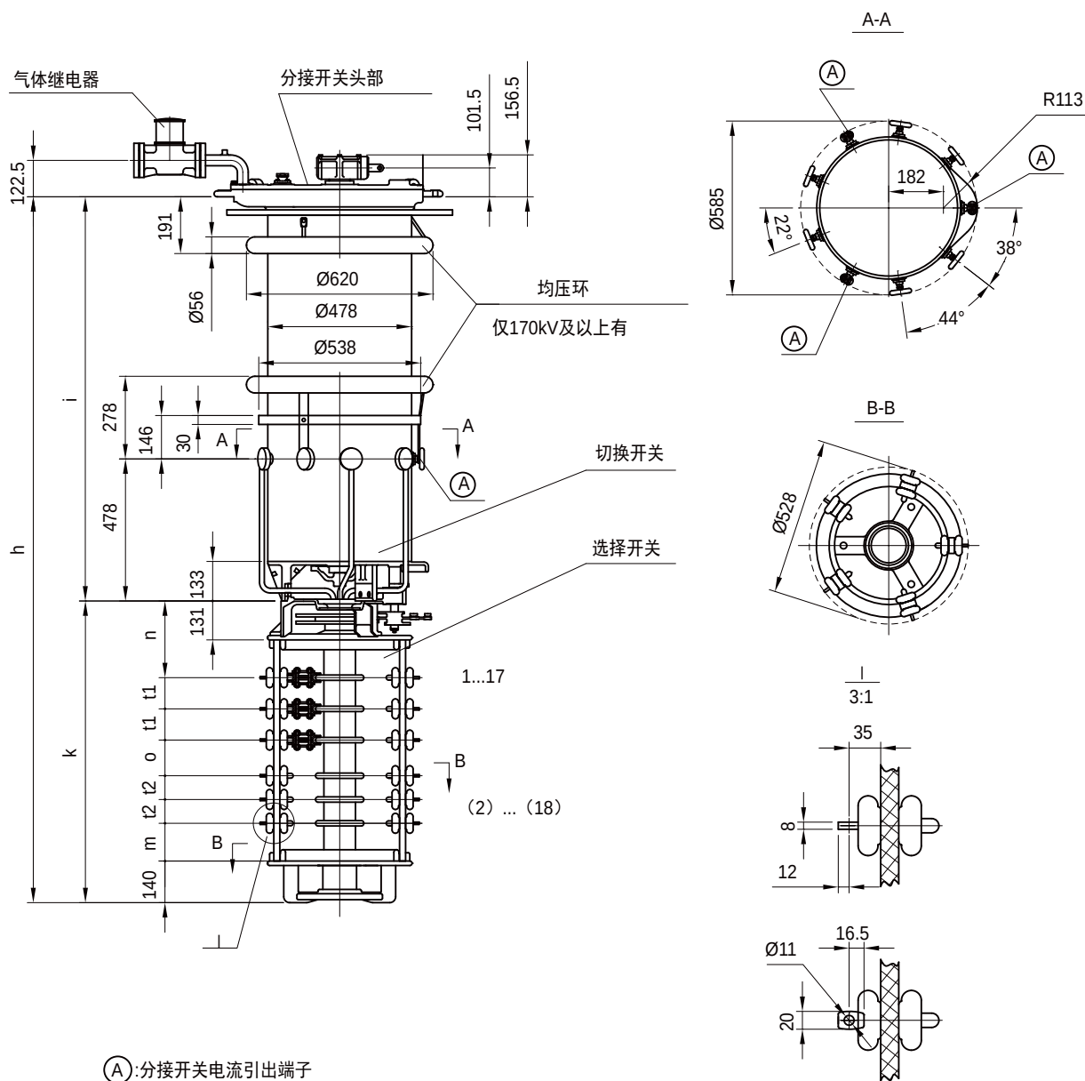
附图 13 CM 型有载开关 I 1200/1500 不带极性选择器
