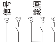
QJ5-25型接线图
