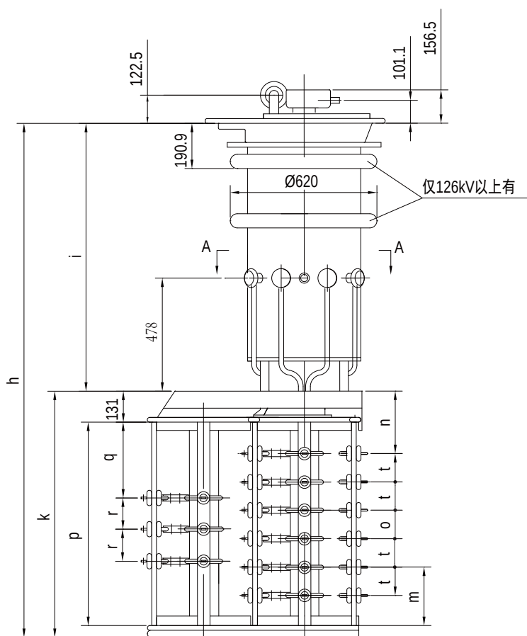
附图38 CM I 1200/1500多级正反调开关外型尺寸图
