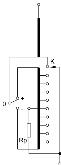
图 8 电位电阻的连接
