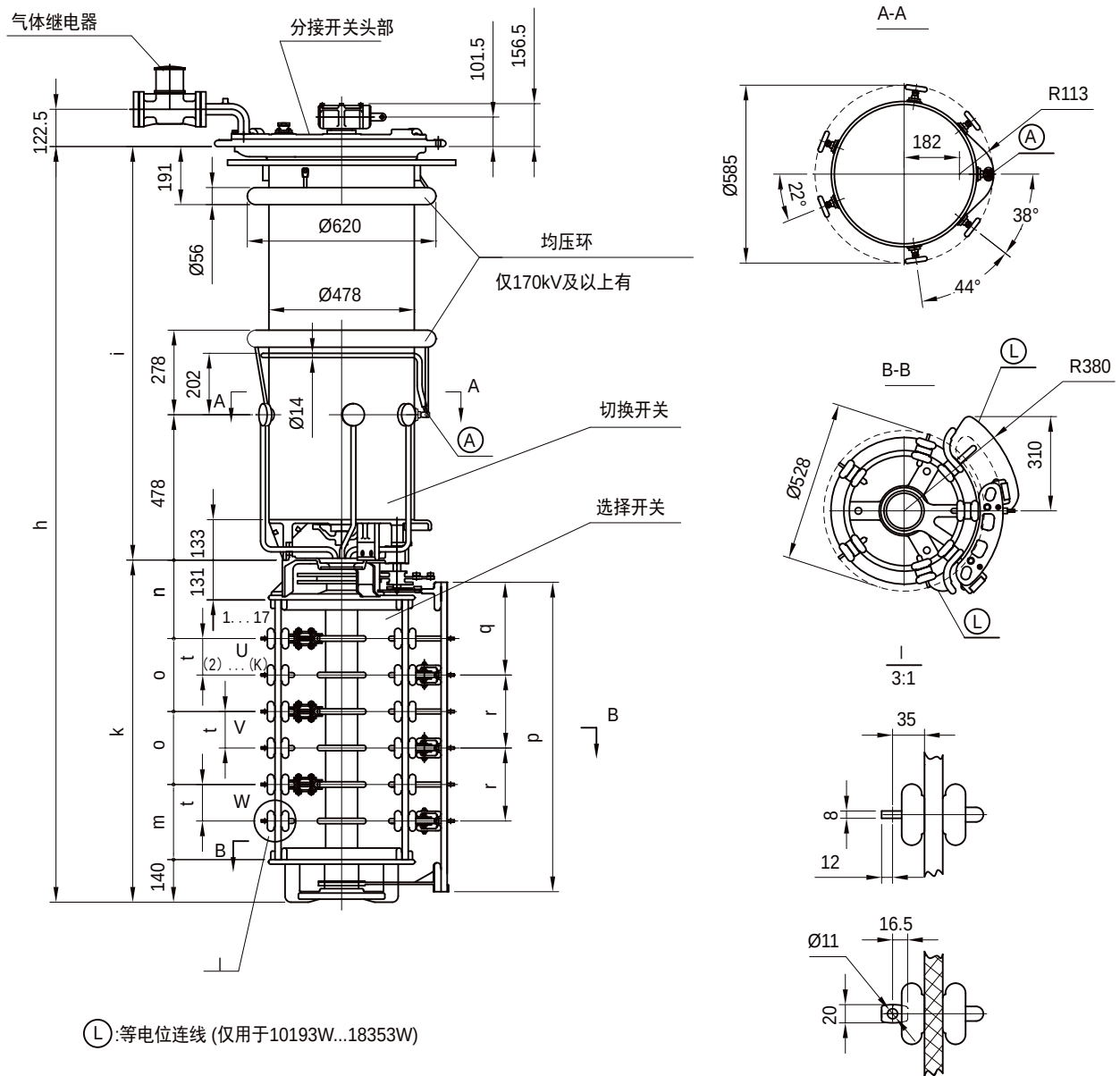
附图 2 CM 型有载开关Ⅲ 500Y/600Y 带极性选择器
