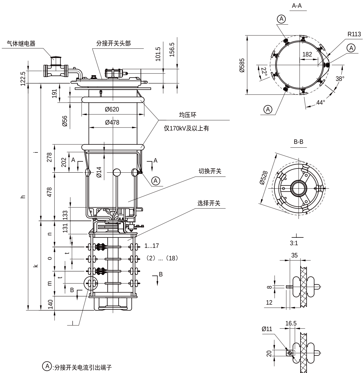
附图 4 CM 型有载开关 II 500/600 不带极性选择器
