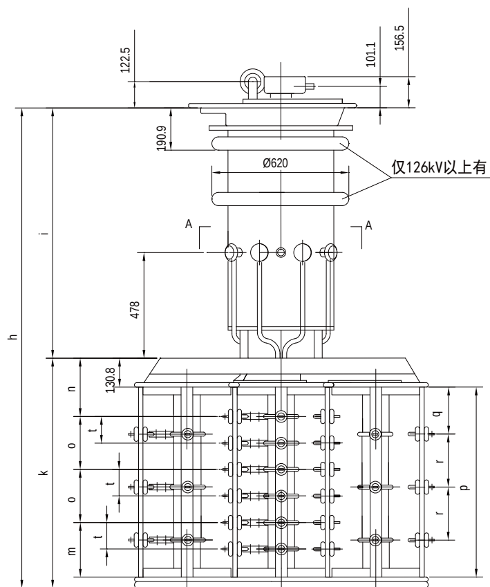
附图 31 CM III 500Y/600Y 多级开关外形尺寸图
