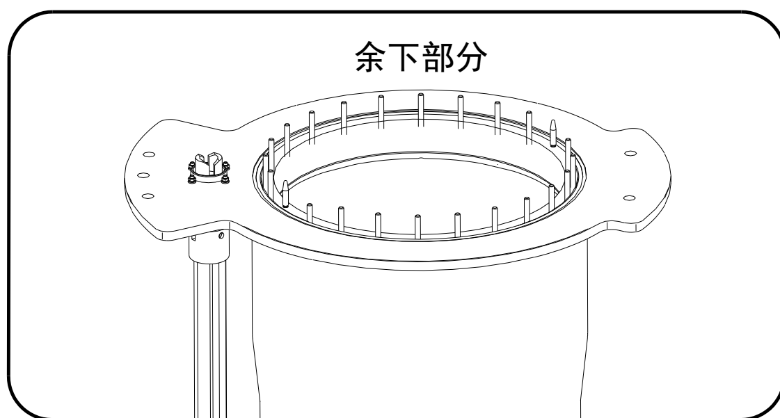
图 5-7 开关安装法兰吊装示意
