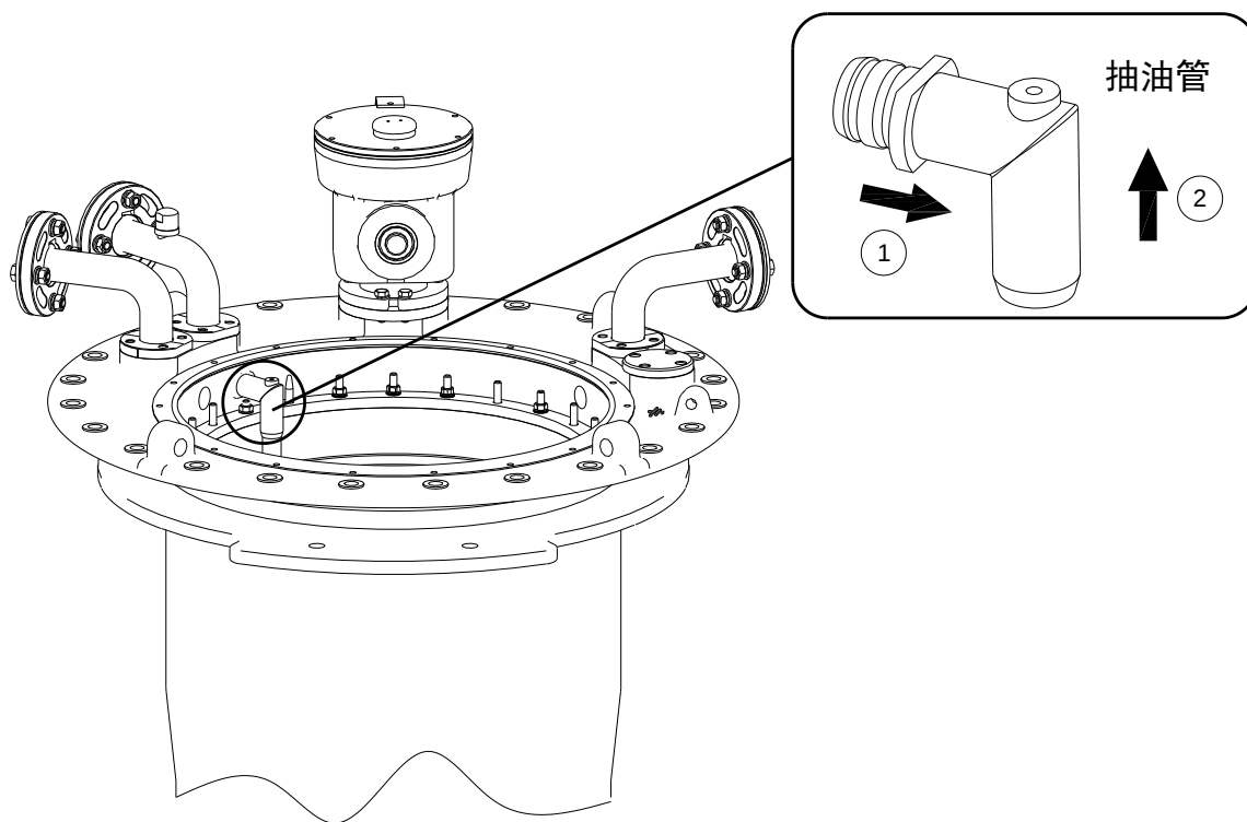
图 5-6 抽油管拆卸示意图
