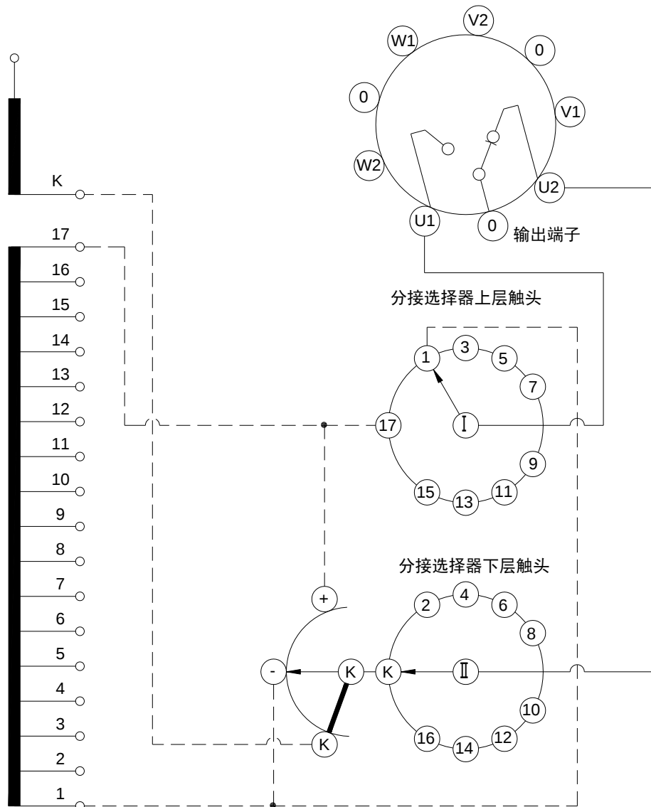
附图 13 CHVT 有载分接开关工作位置表和接线原理图 18353W(L)
