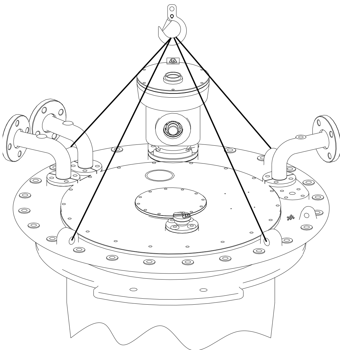
图 4-5 开关吊装图
