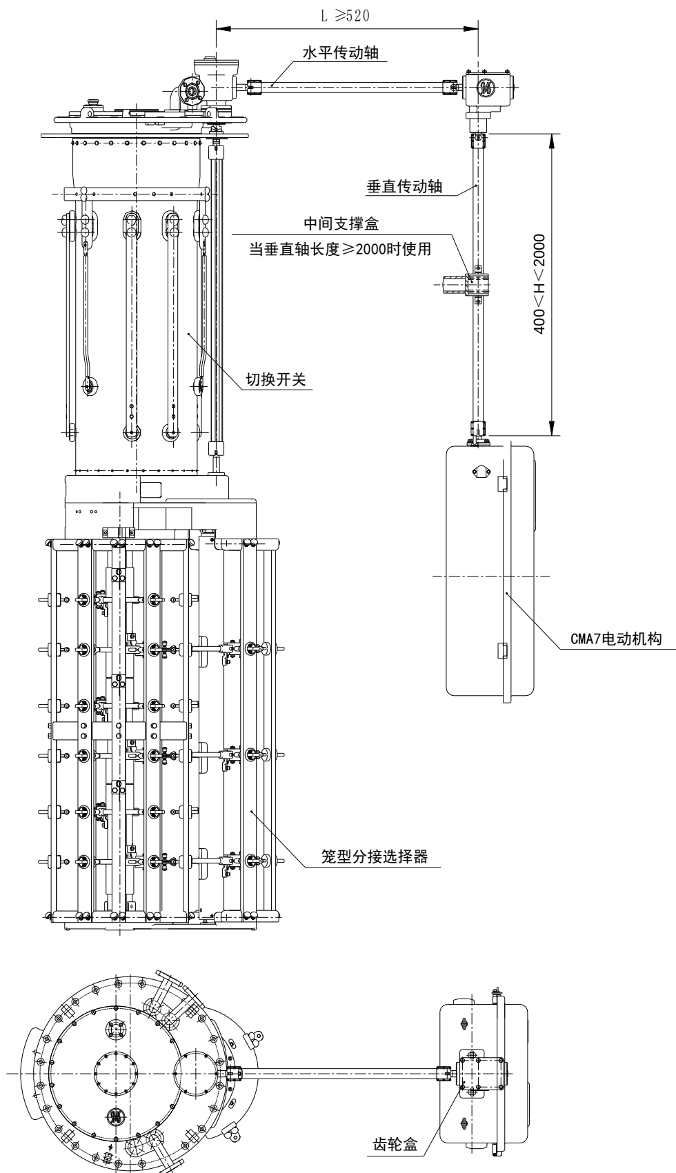
附图 6 CHVT 分接开关与 CMA7 电动机构连接布置图
