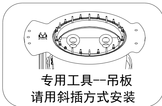
图 5-8 选择器定位板，开关油室起吊环
