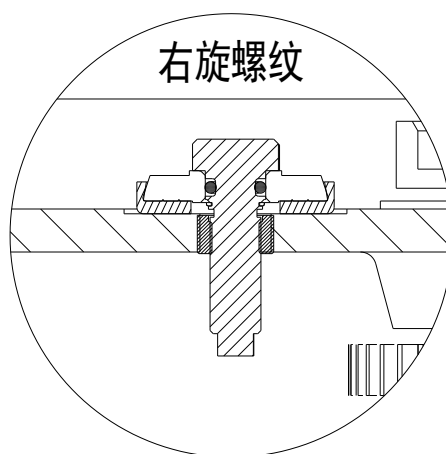
局部放大剖切图 (逆时针松开)
