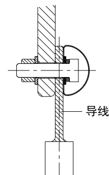
剖切图
