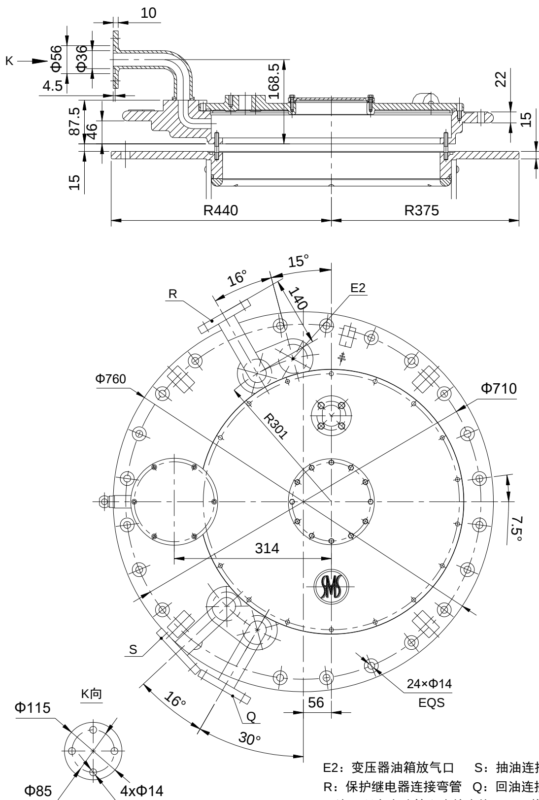
附图 1 CHVT 有载分接开关变压器安装法兰尺寸
